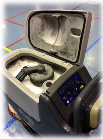
Figure 8 Slå av strøm, og dermed vakum, Åpne lokk for å sjekke om avfallsvannstanken er full
